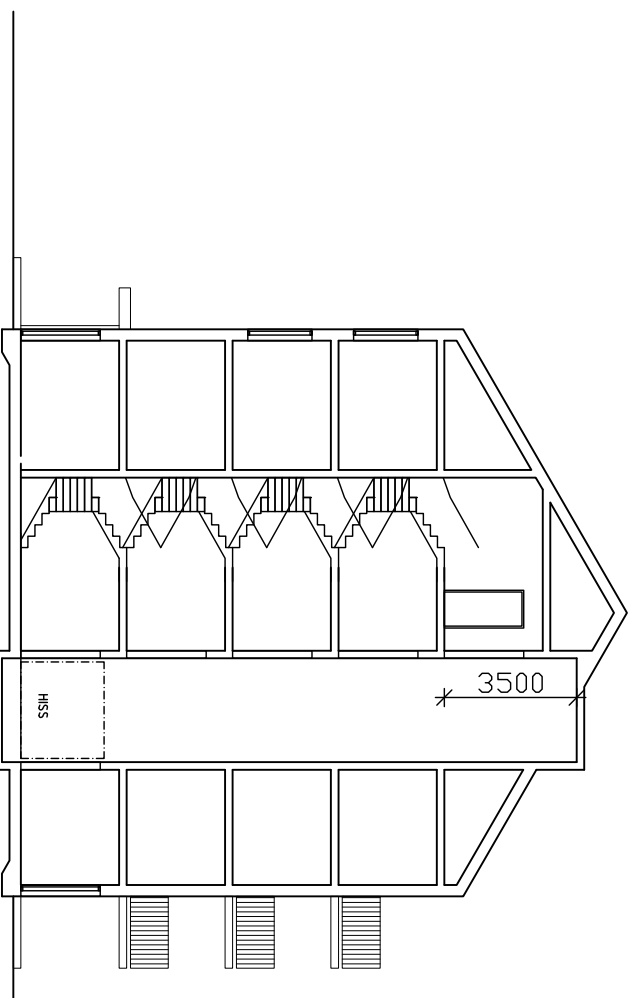
SEKTION A-A
