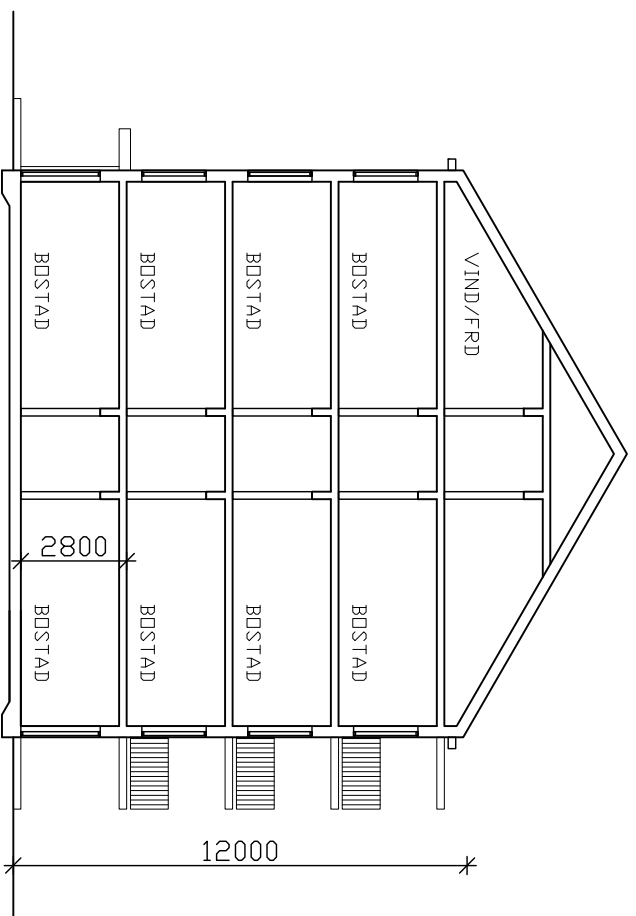
SEKTION B-B
