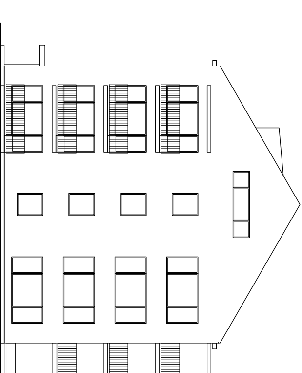
FASAD SIDA
