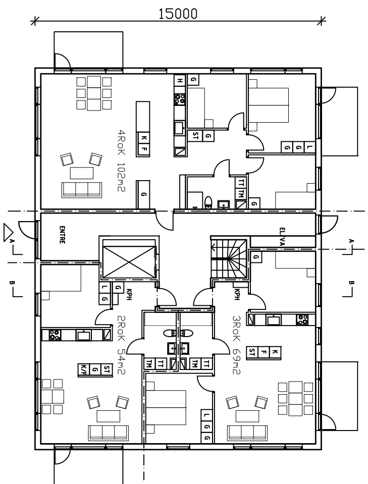
ENTREPLAN PLAN 1
