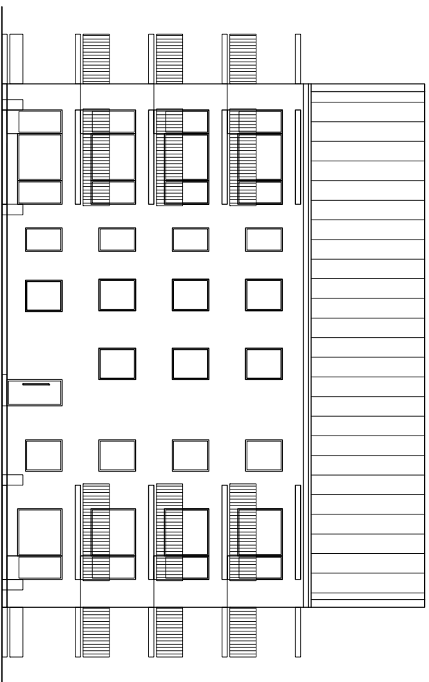
FASAD GÅRDSIDA
